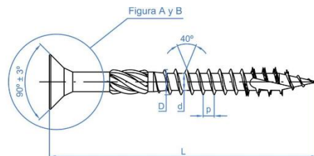
Figura A: avellanado interior 2.5 + 4.5
