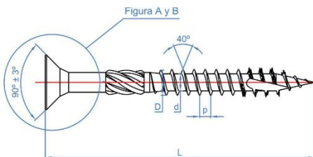
Figura A: avellanado interior para Ø2.5 ÷ Ø4.5
