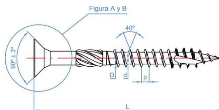
Figura A: avellanado interior 4.0 + 4.5
